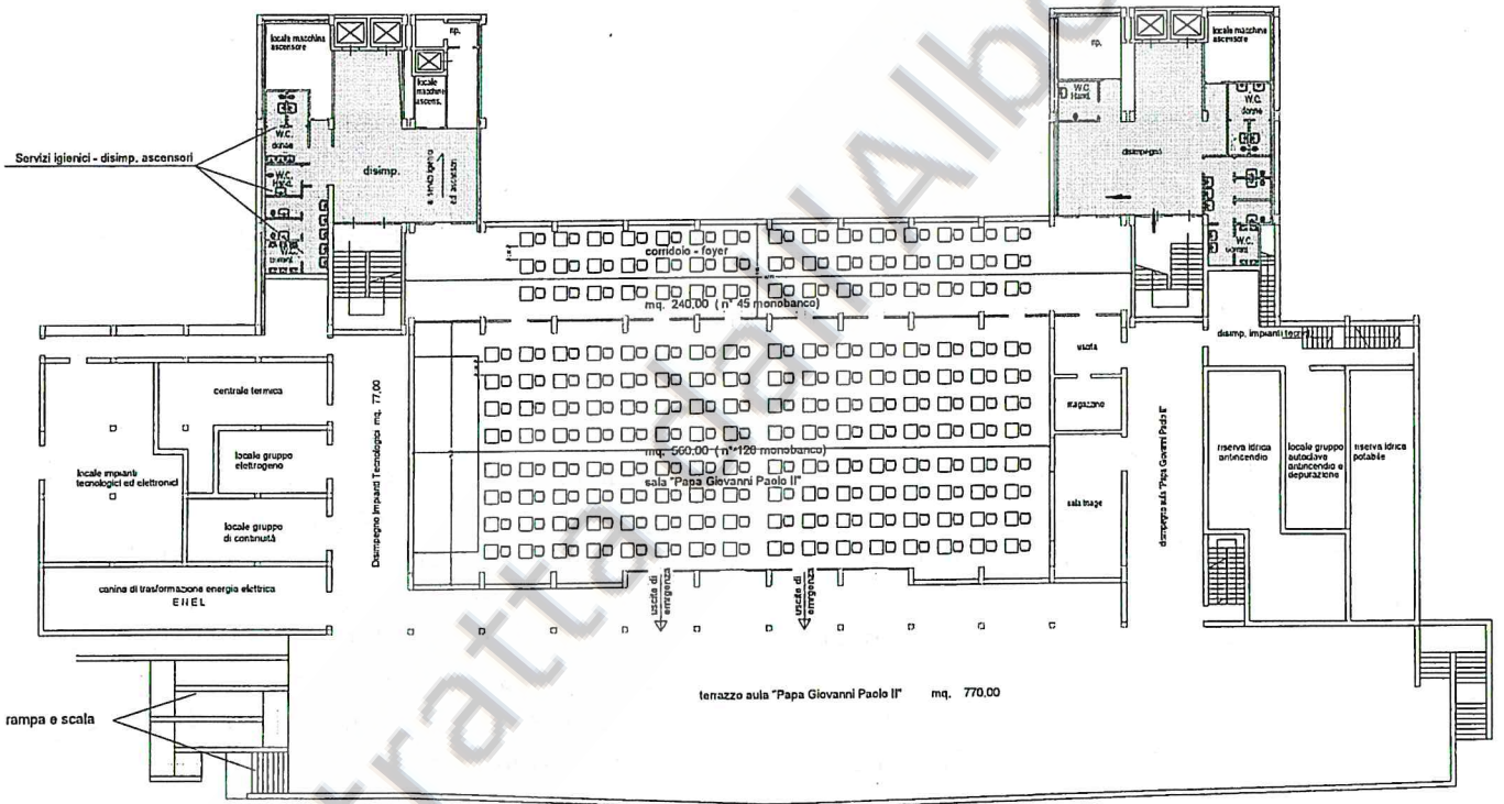
PIANTA PIANO -2 (2° Seminterrato)
