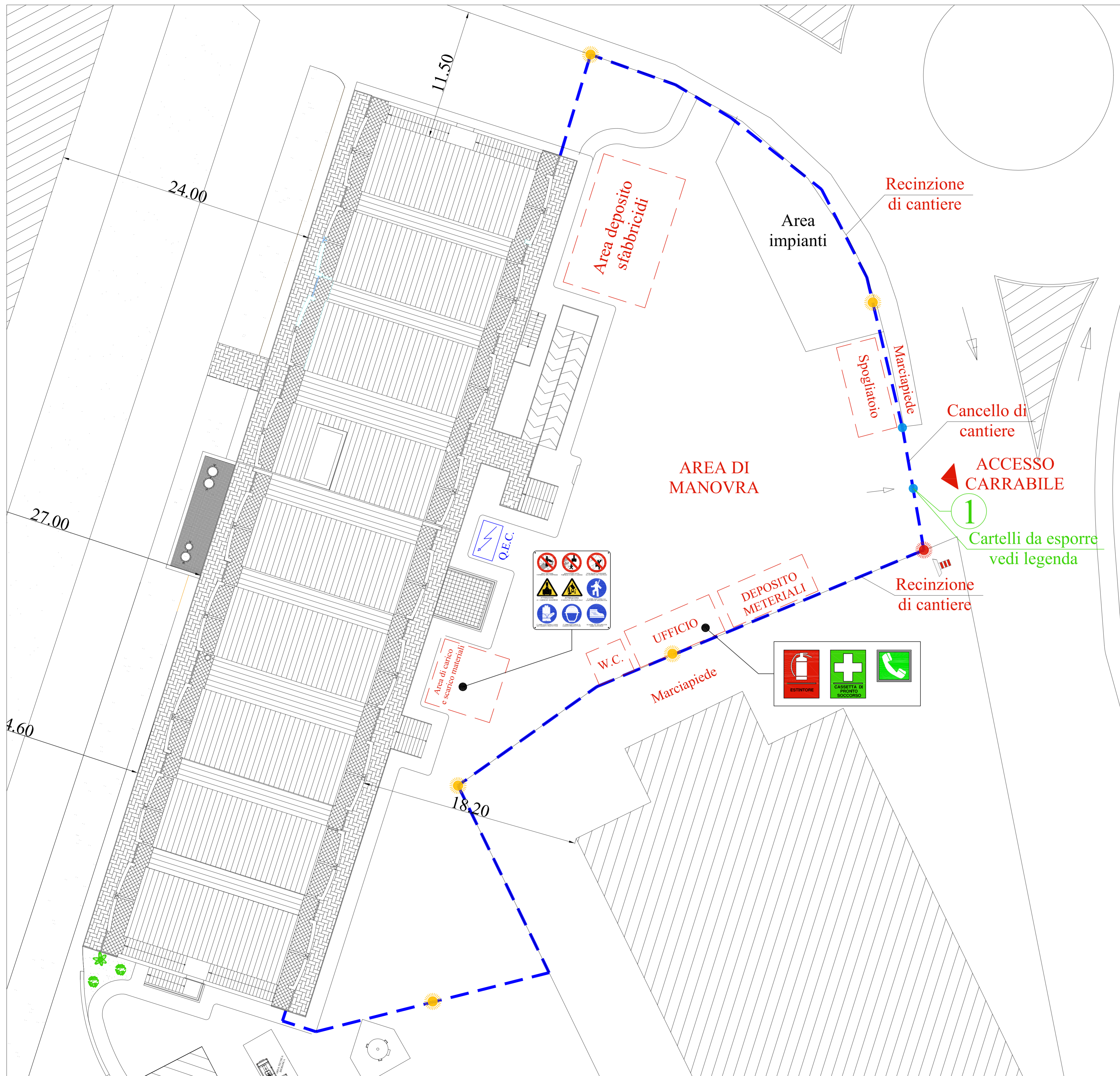
PLANIMETRIA - AREE DI CANTIERE
