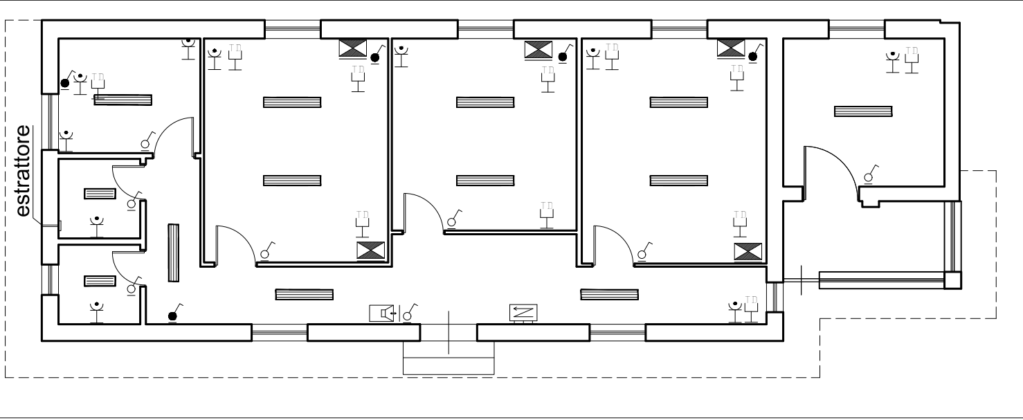
SCHEMA IMPIANTO ELETTRICO E DI ILLUMINAZIONE
