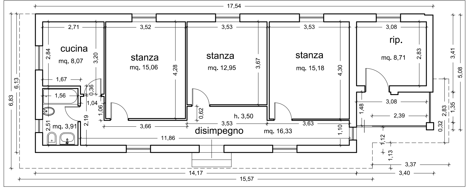
PLANIMETRIA STATO ATTUALE
