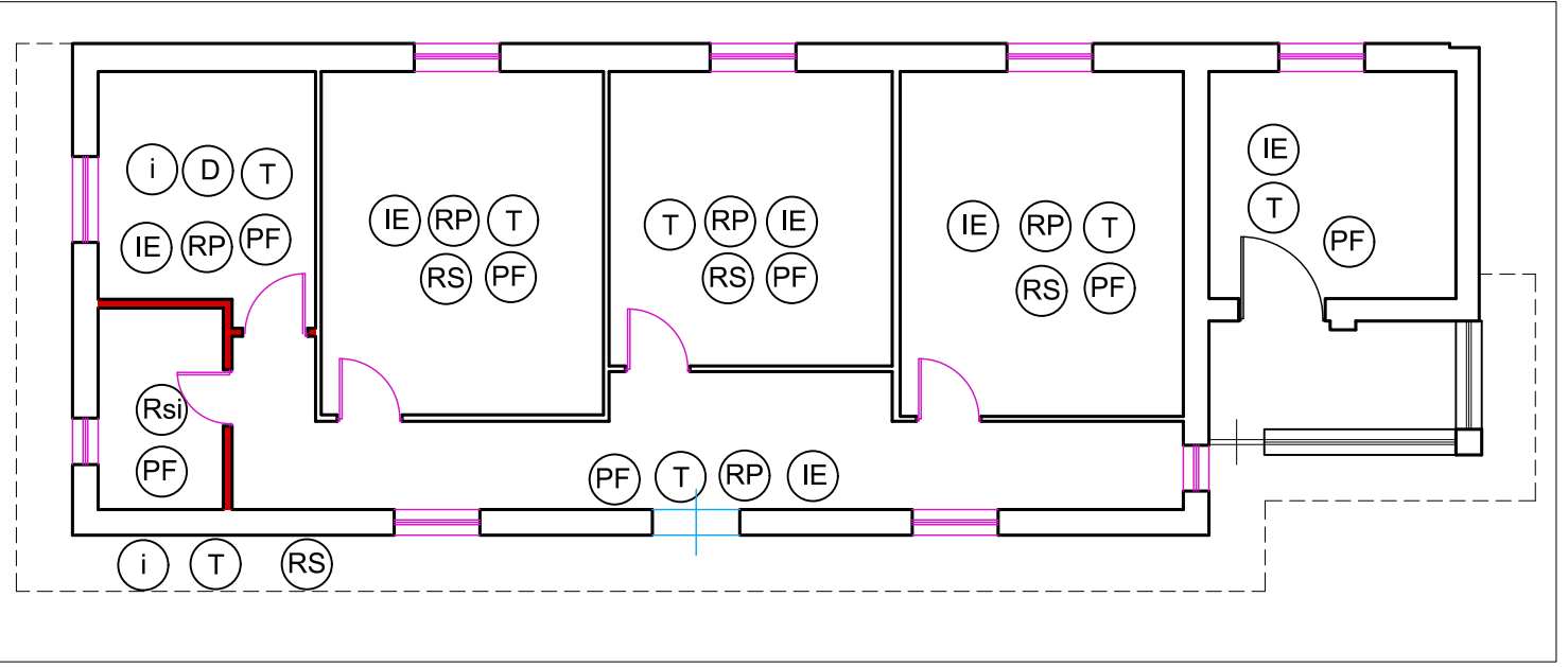
PLANIMETRIA DELLE DEMOLIZIONI E DEGLI INTERVENTI
