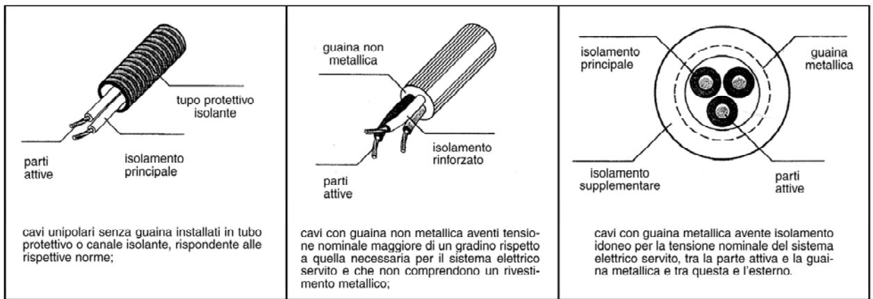
FIG. 6 - Cavi a doppio isolamento. Tipologie
