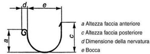
FIG. 5 - Canale di gronda - Tipo
